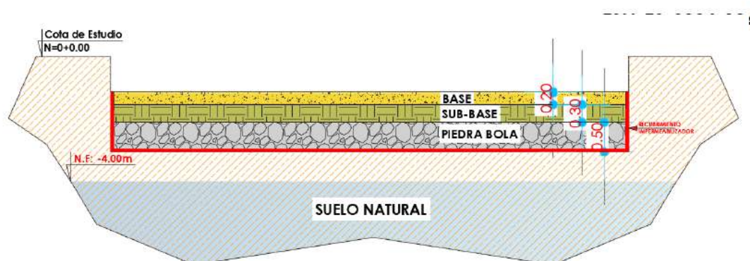
Ilustración 9 Solución Constructiva estructuras de un nivel. Fuente: Propia.
